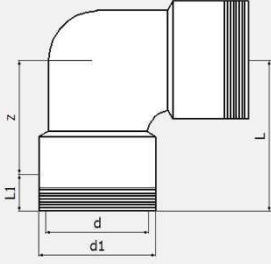
HDPE ELEKTROFÜZYON DİRSEK 90° PN16 / SDR 11 HDPE EF ELBOW 90° PN16 / SDR 11
