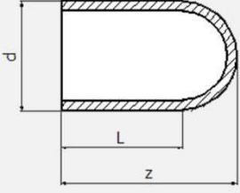
HDPE ENJEKSİYON KÖR TAPA PN16 / SDR 11 HDPE INJECTED END CAP PN16 / SDR 11
